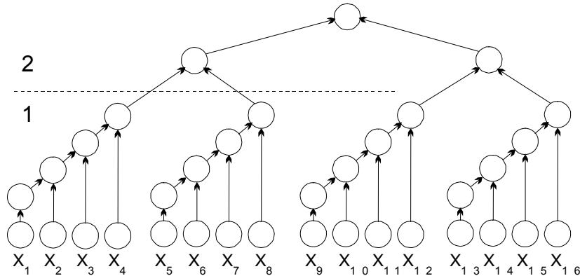
Рис. 2.4. Модифицированная каскадная схема суммирования
