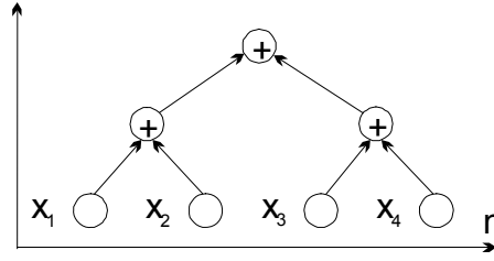
Рис. 2.3. Каскадная схема алгоритма суммирования
